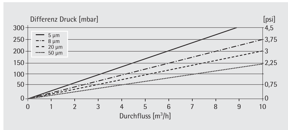
Wasserdurchfluss 10" Filterkerze
